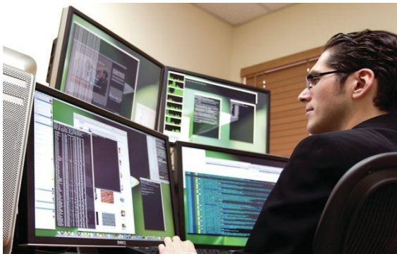
IT- менеджеры
